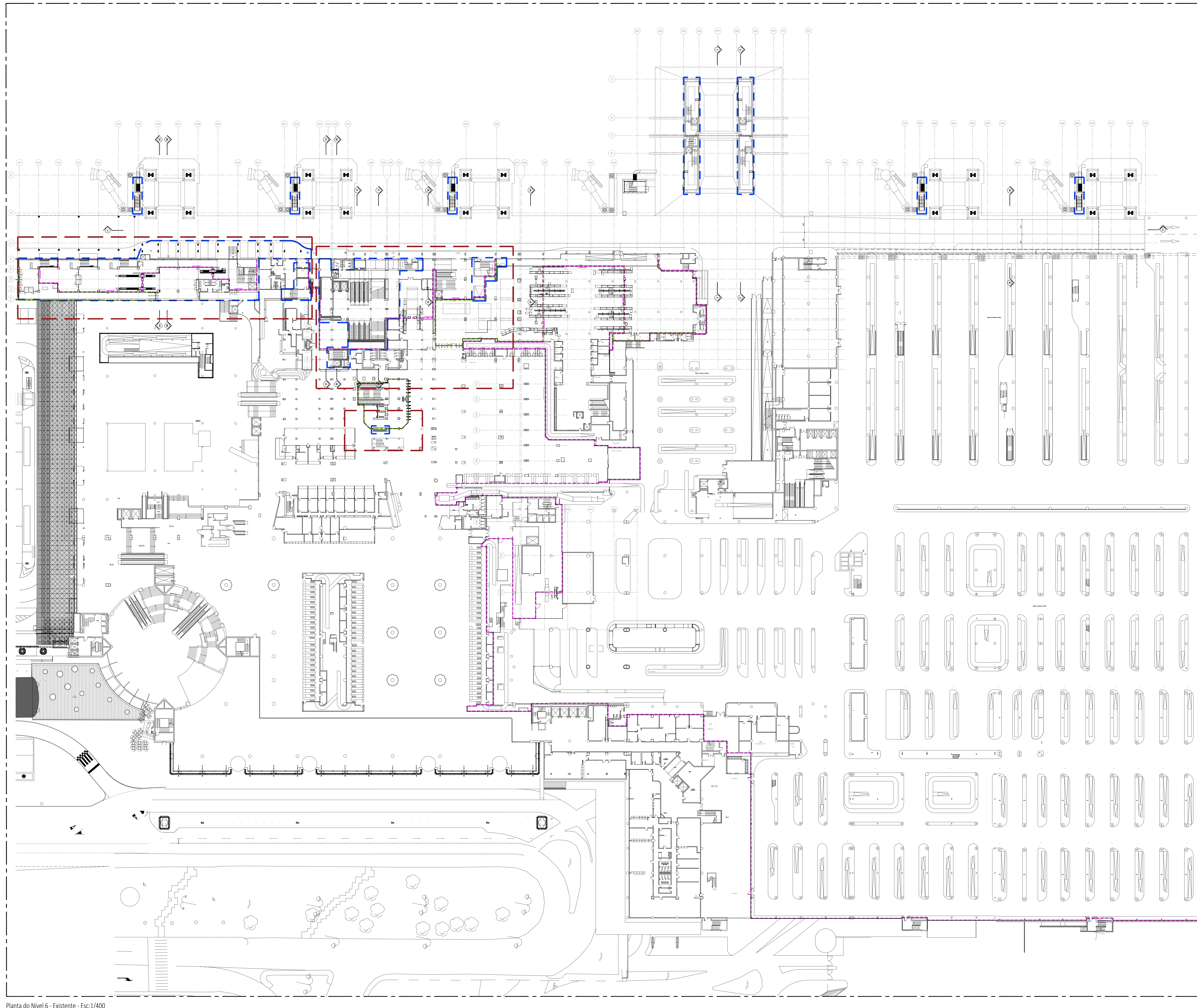
Planta do Nível 6 - Existente - Esc:1/400
