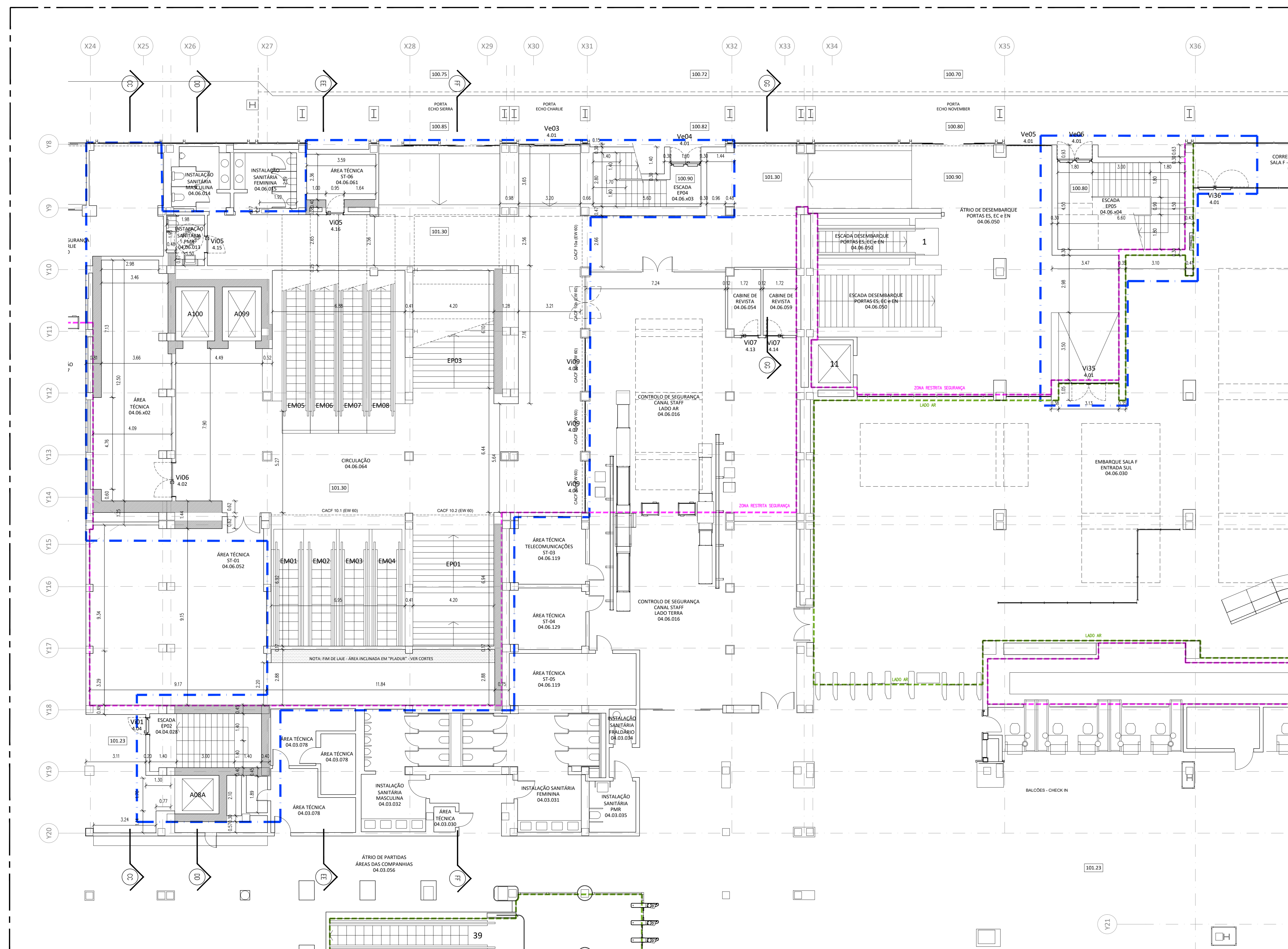
Planta do Nível 4 - Proposta - Esc:1/100
