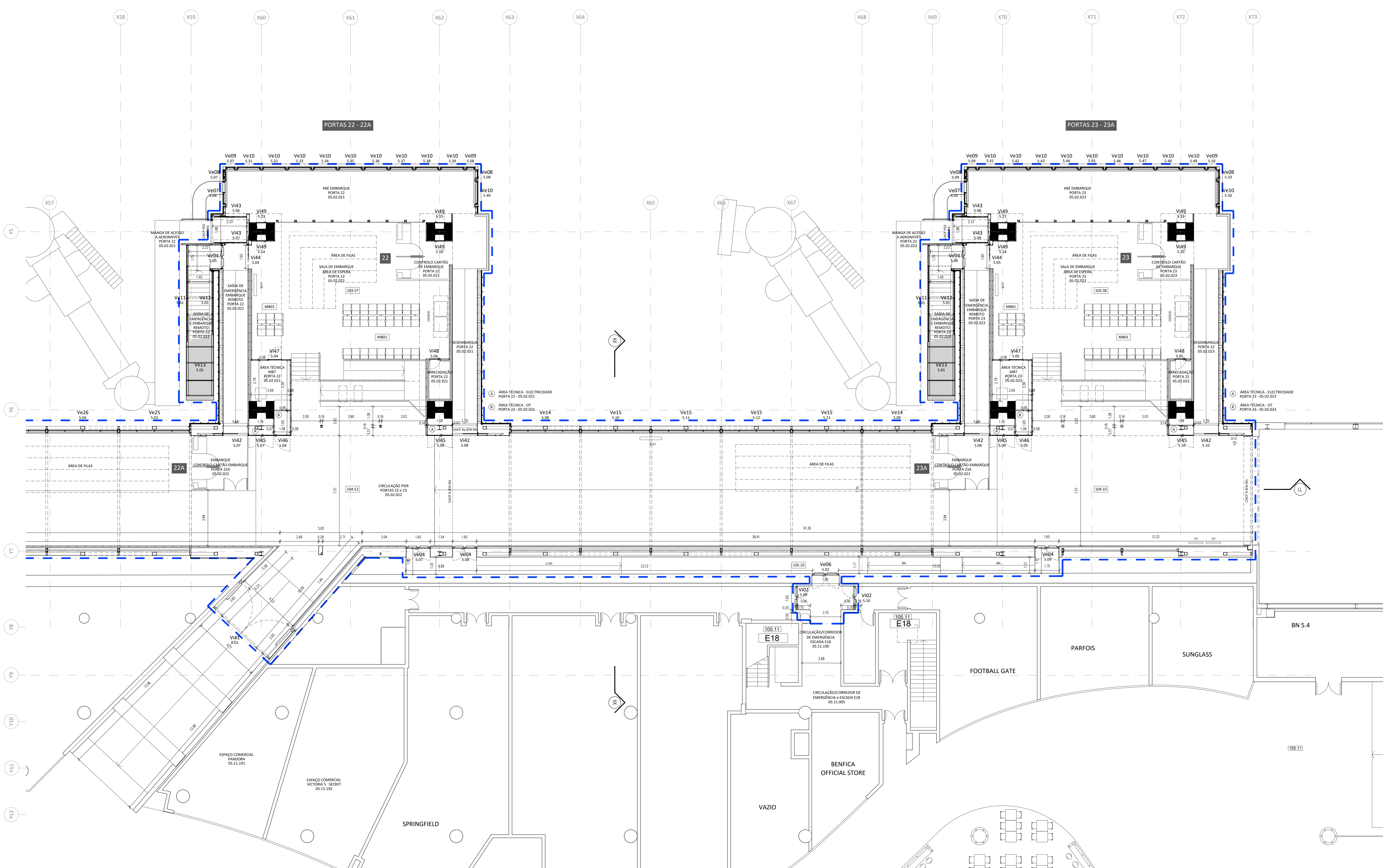
Planta do Nível 5 - Zona D - Proposta - Esc:1/100
