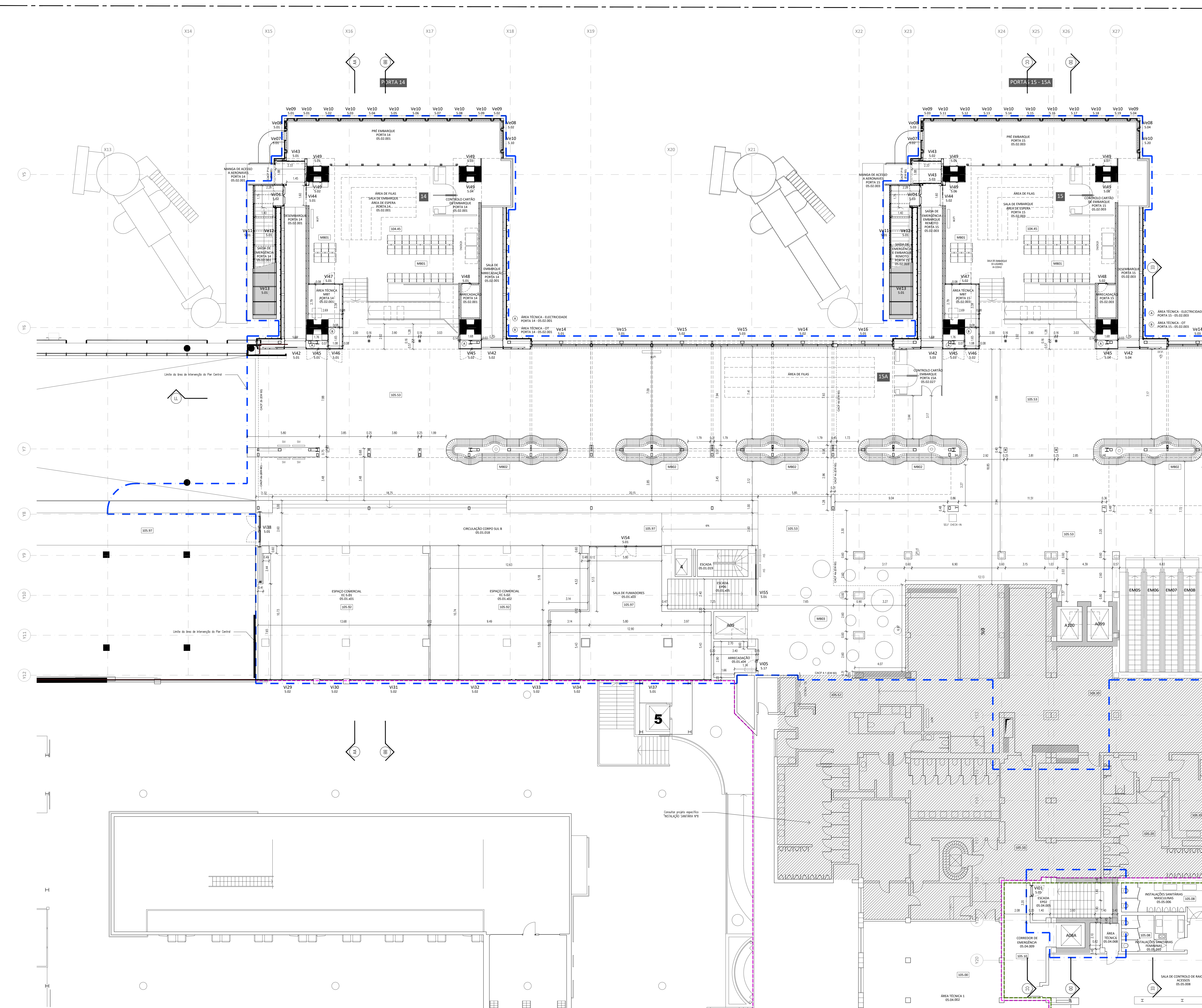
Planta do Nível 5 - Zona A - Proposta - Esc:1/100
